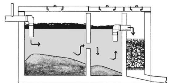
Schéma d'un type de fosse septique
