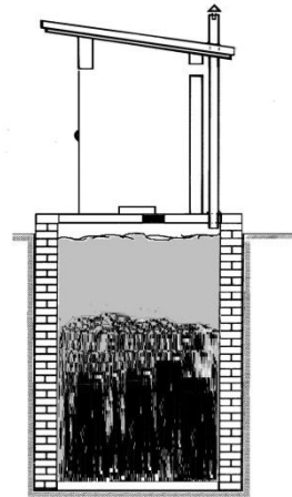
Schéma d'une fosse simple
