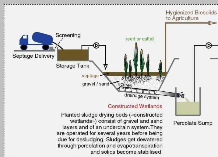
Station à lits de séchage plantés proposée pour Nam Dinh
