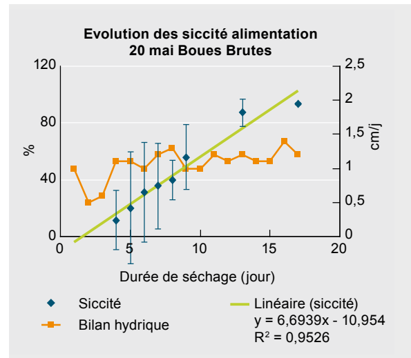
Figure 7 : Evolution siccité et évaporation en fonction du temps (alimentation du 20 Mai).
