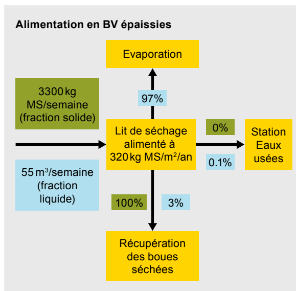
Figure 5 : Bilans massique et volumétrique des MS et de l'eau respectivement.
