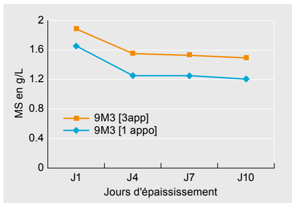
Figure 5 : Variation des MS en fonction du mode de fractionnement des charges
