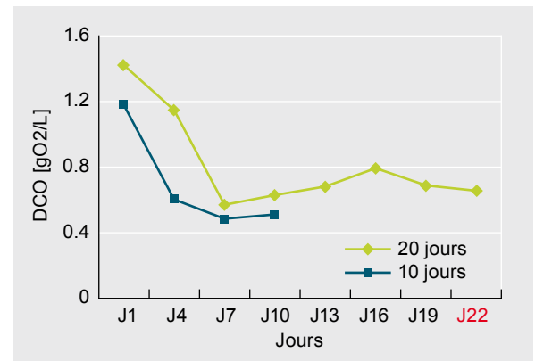
Figure 6 : Evolution de la DCO en fonction de la durée de l'épauississement avec 9 m 3 apport unique
