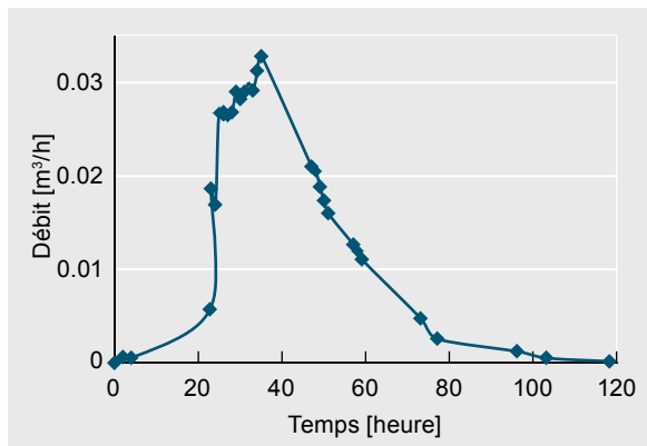
Figure 2 : Variation de débit d'infiltration en fonction du temps, alimentation du 30 Juin.
