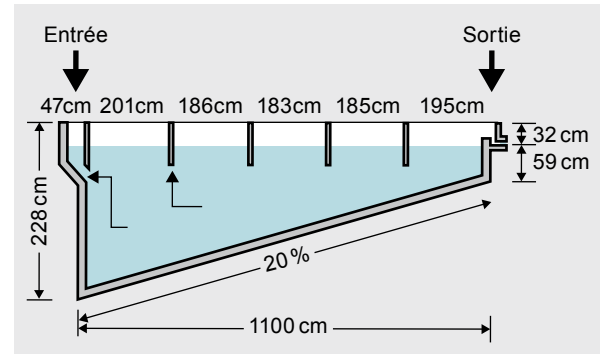
Figure 1: Vue schématique du décanteur épaisseur
