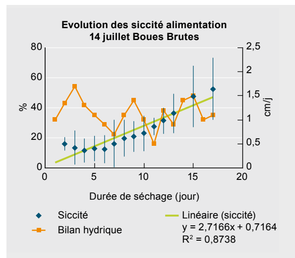
Figure 8 : Evolution siccité et évaporation en fonction du temps (alimentation du 14 Juillet).
