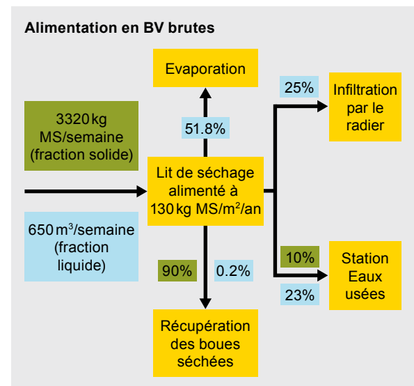
Figure 9 : Dispatching des charges massique et volumétrique autour d'un lit de séchage.
