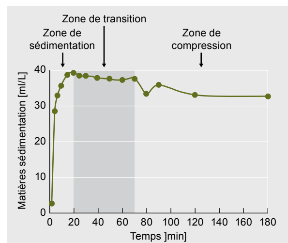
Figure 2: Courbe d'évolution des matières décantables.
