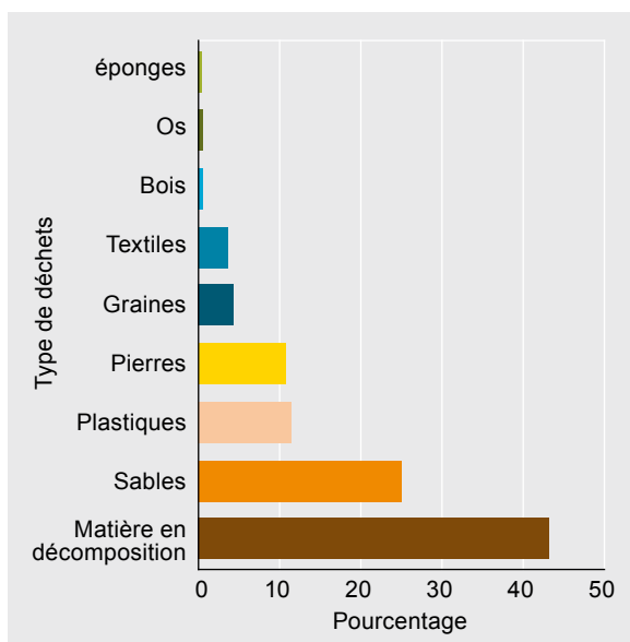
Figure 3: Pourcentage massique des différentes classes de déchets
