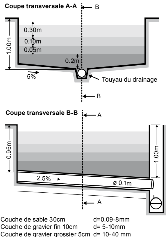
Figure 1 : Présentation de la constitution des lits en coupe
