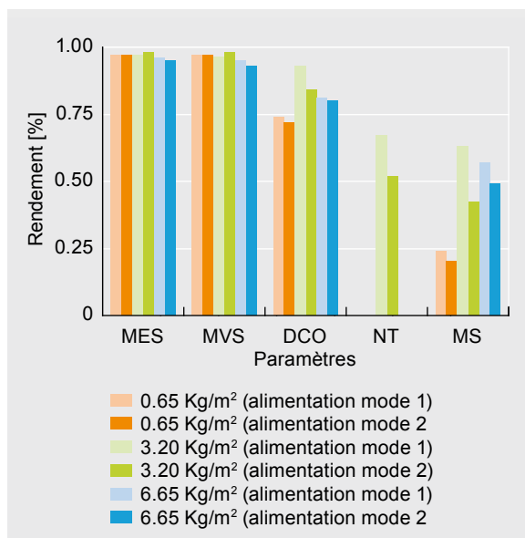
Figure 4 : Rendement épuratoire des lits en fonction de la charge
