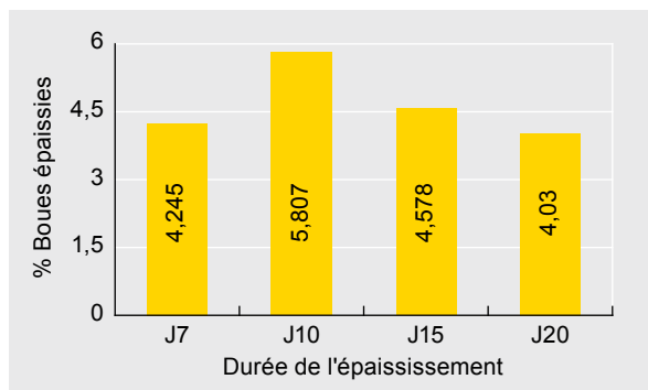
Figure 7 : Pourcentage de boues épaissies en fonction de la durée de l'épaississement
