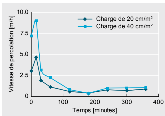
Figure 2 : Évolution de la vitesse de percolation en fonction de la charge hydraulique.
