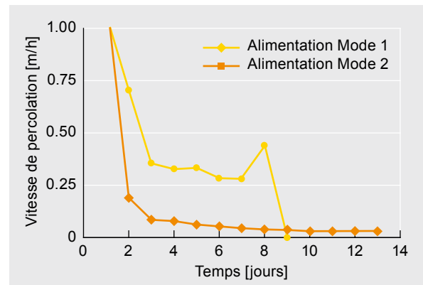
Figure 3 : Évolution de la vitesse de percolation en fonction du mode d'alimentation
