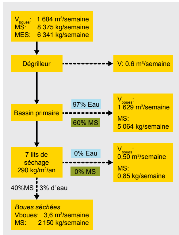
Figure 6 : Résumé schématique du dispatching des différents flux de matières
