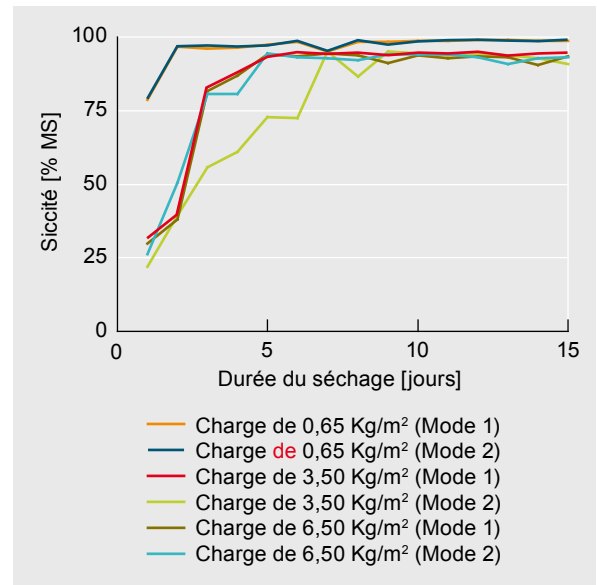
Figure 6 : Évolution de la siccité en fonction de la charge
