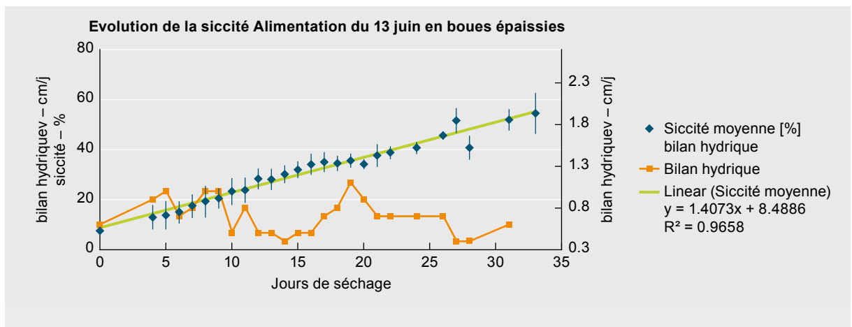
Figure 3 : Evolution du séchage moyen en fonction du temps de l'alimentation du 13 Juin.
