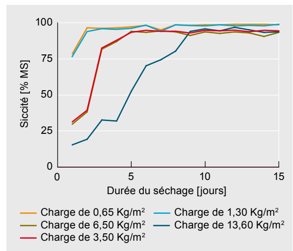
Figure 7 : Évolution de la siccité en fonction du mode d'alimentation
