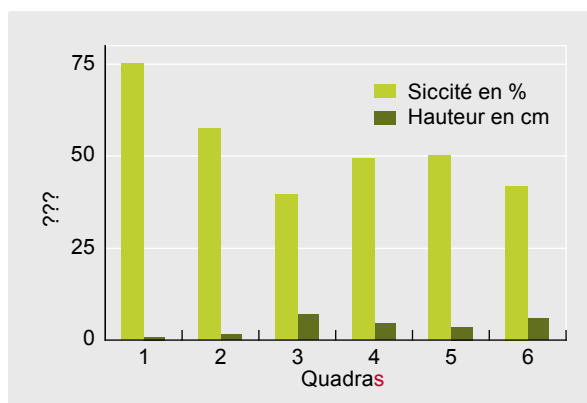
Figure 1 : Hauteur et siccité des boues déshydratées
