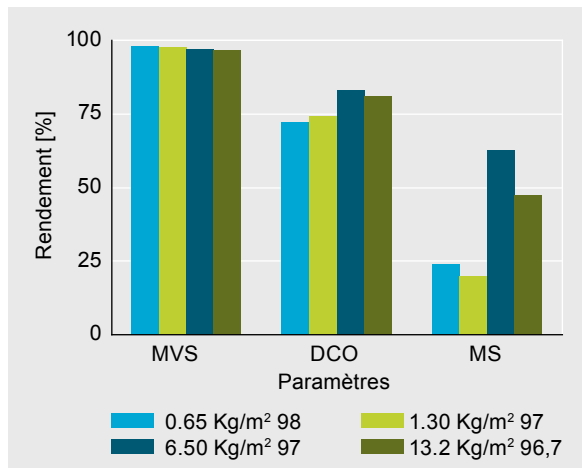
Figure 5: Rendement épuratoire des lits en fonction du mode d'alimentation
