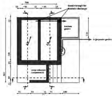
Module "Urine-Separation Vermitoilet" (cont.)
